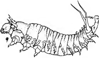
Fig. 345. Cassida nebulosa L.
